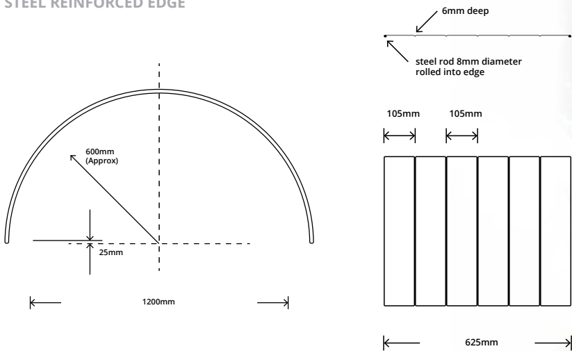
STEEL REINFORCED EDGE
